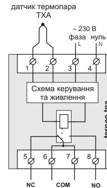
Схема 1. Спрощена внутрішня схема та схема підключення
