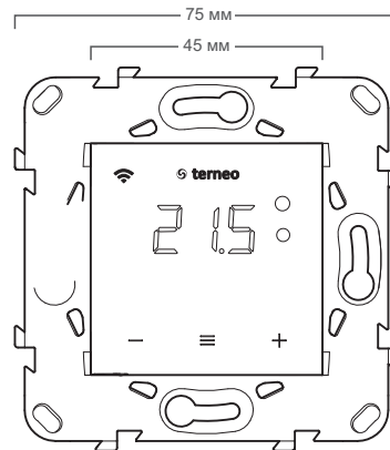
Рисунок 1. Габаритні розміри
