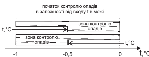
Рисунок 4. Мінімальні межі з гістерезисом > 1 °C.
