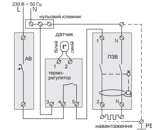
Схема 2. Підключення автоматичного вимикача і ПЗВ
