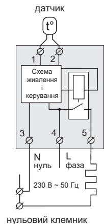
Схема 1. Спрощена внутрішня схема і схема підключення
