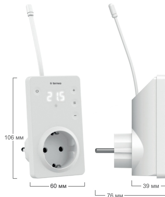
Рисунок 1. Габаритні розміри terneo srz
